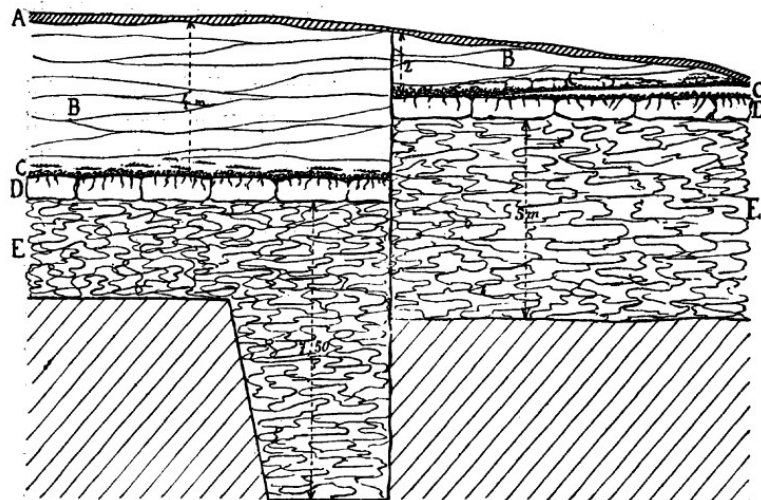
Coupe de l'exploitation de phosphate de M. Passelecq, au Sud de Ciplly.
